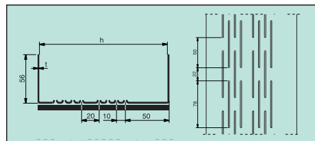
SKYP Vnější stěnový vodící profil s izolací
